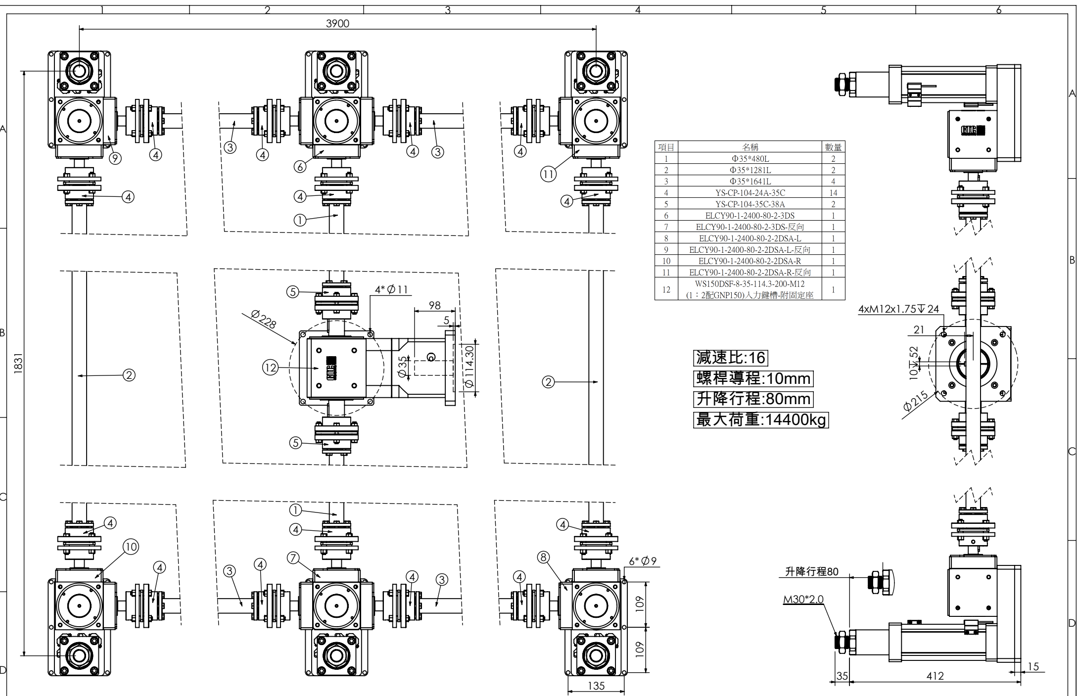
圖名 ELCY90-7-14400-80-16-35-114.3-200-M12(1831 * 3900) GTC 鼎億自動化股份有限公司 Gumptious technology Co.
